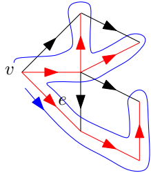
\vec{T} \cap \vec{T}^*
